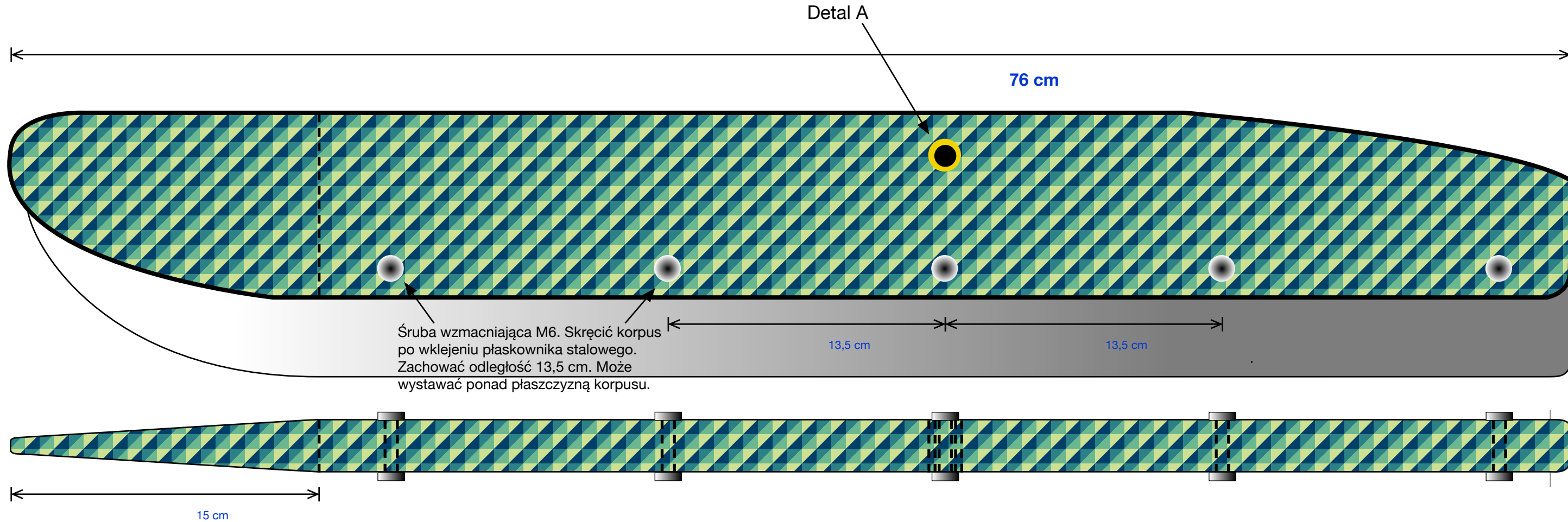
Przykładowe rozwiązanie śruby wzmacniającej korpus
